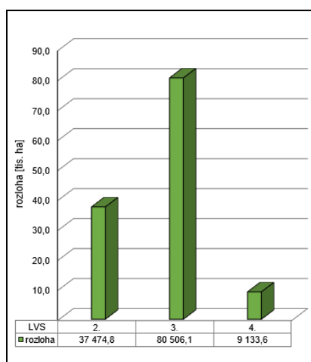
Obr. 15: Zastoupení LVS v PLO 6
