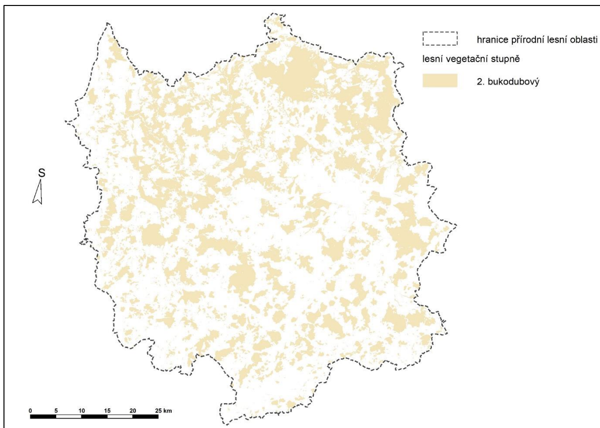
Obr. 3: Prostorová lokalizace transformovaných LVS v PLO 6 dle scénáře HadGem varianty RCP 45 v období E a varianty RCP 85 v obdobích C, D
