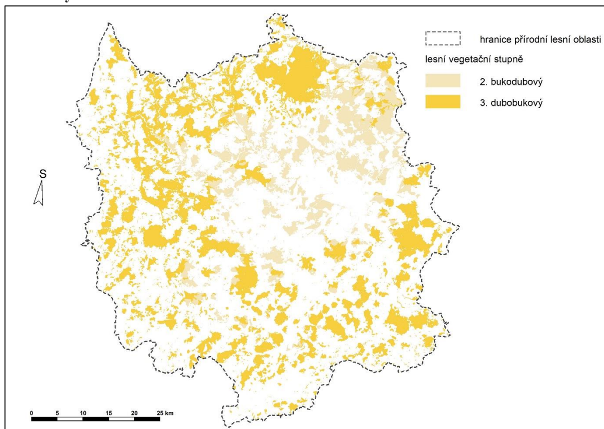
Obr. 1: Prostorová lokalizace transformovaných LVS v PLO 6 dle scénáře HadGem varianty RCP 45 v období C
