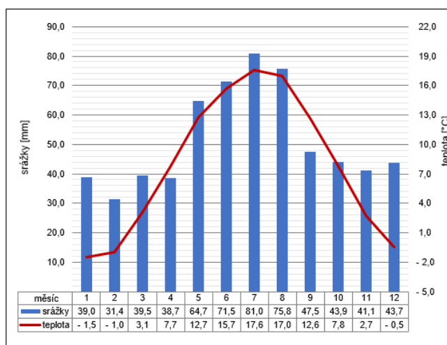
Obr. 14: Klimadiagram pro 3. LVS
