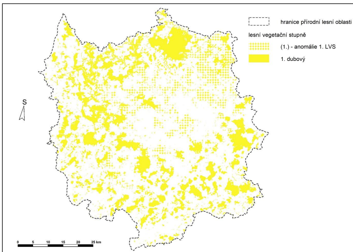
Obr. 4: Prostorová lokalizace transformovaných LVS v PLO 6 dle scénáře HadGem varianty RCP 85 v období E
