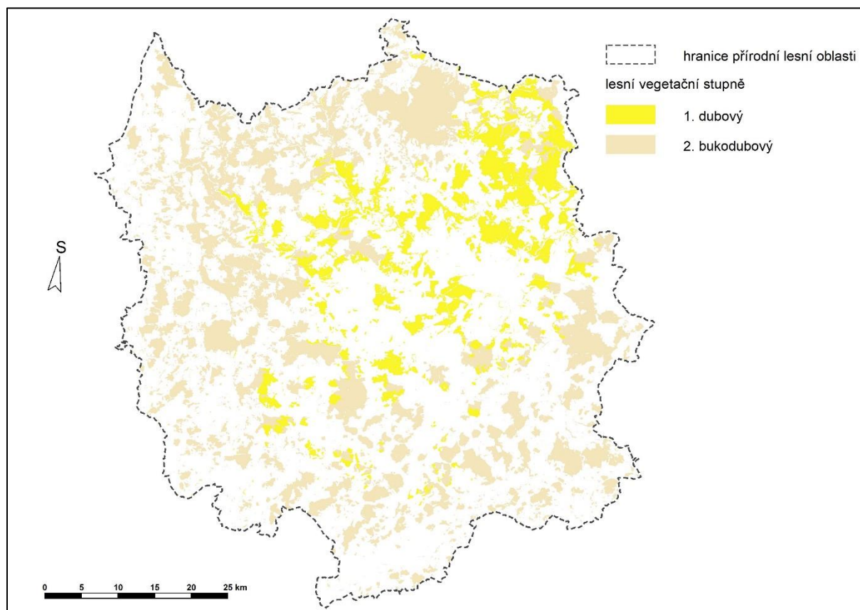
Obr. 2: Prostorová lokalizace transformovaných LVS v PLO 6 dle scénáře HadGem varianty RCP 45 v období D
