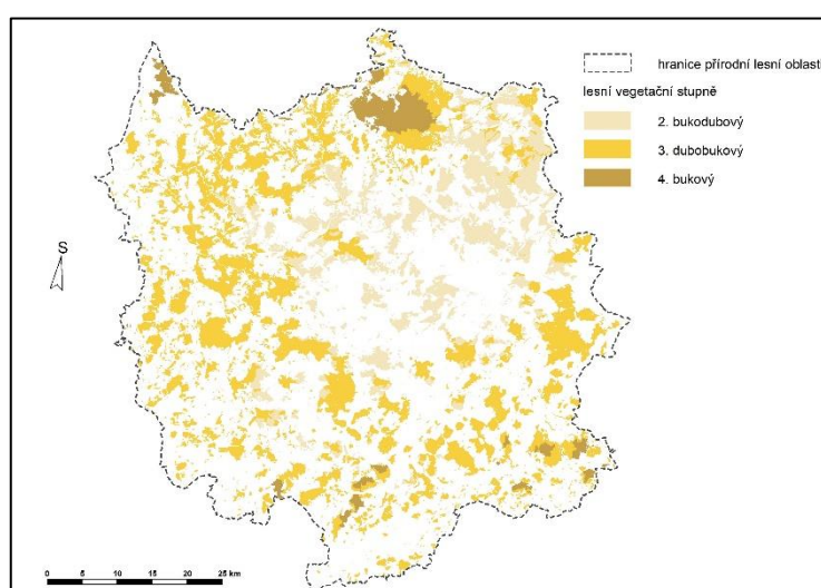
Obr. 16: Prostorová lokalizace LVS v PLO 6
