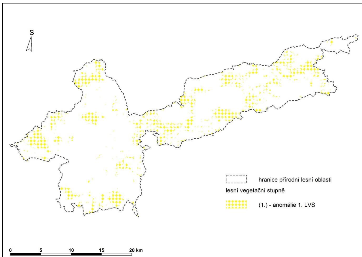
Obr. 2: Prostorová lokalizace transformovaných LVS v PLO 2a dle scénáře HadGem varianty RCP 85 v období E
