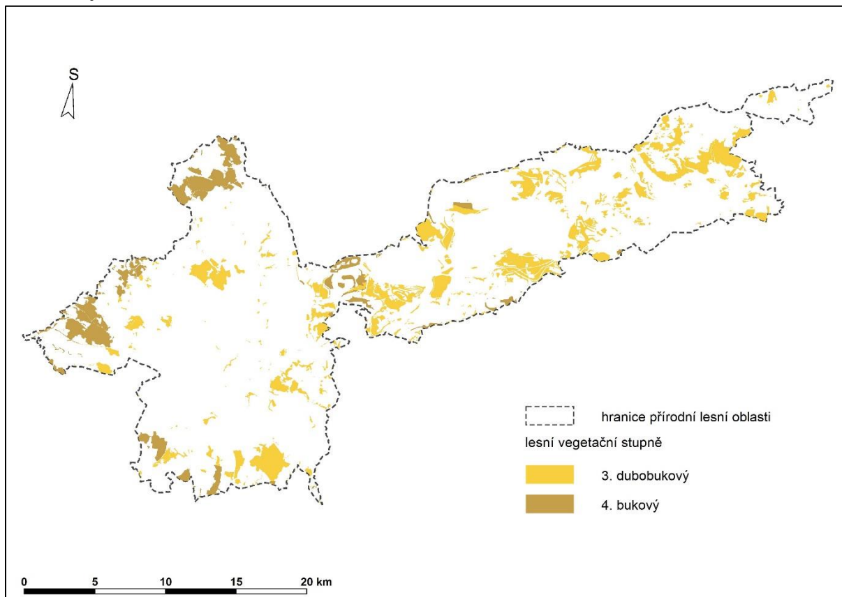
Obr. 1: Prostorová lokalizace transformovaných LVS v PLO 2a dle scénáře HadGem varianty RCP 45 i 85 v období C
