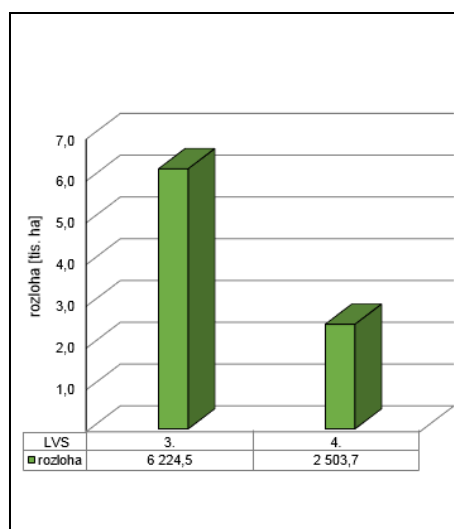
Obr. 15: Zastoupení LVS v PLO 2a
