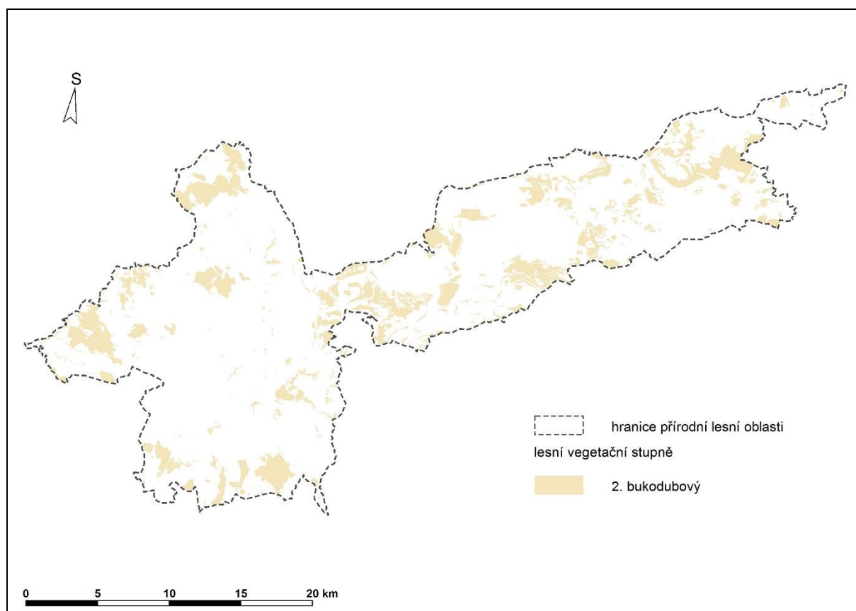
Obr. 3: Prostorová lokalizace transformovaných LVS v PLO 2a dle scénáře HadGem varianty RCP 45 v obdobích D, E a varianty RCP 85 v období D
