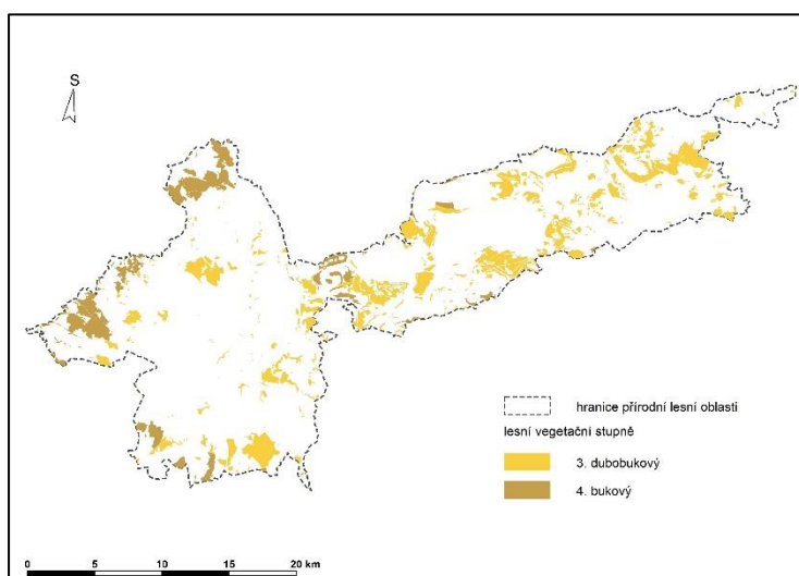
Obr. 16: Prostorová lokalizace LVS v PLO 2a
