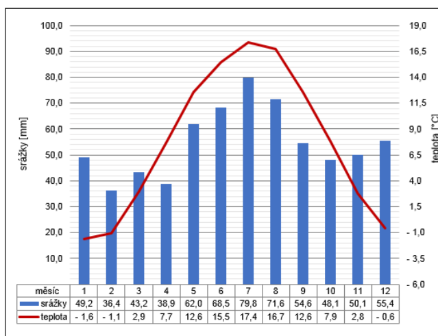
Obr. 14: Klimadiagram pro 4. LVS
