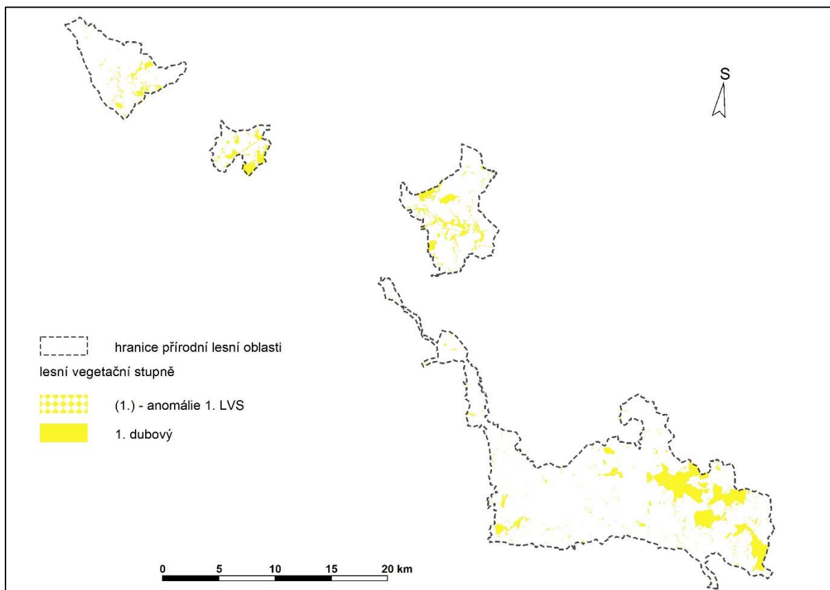
Obr. 2: Prostorová lokalizace transformovaných LVS v PLO 32 dle scénáře HadGem varianty RCP 85 v období E
