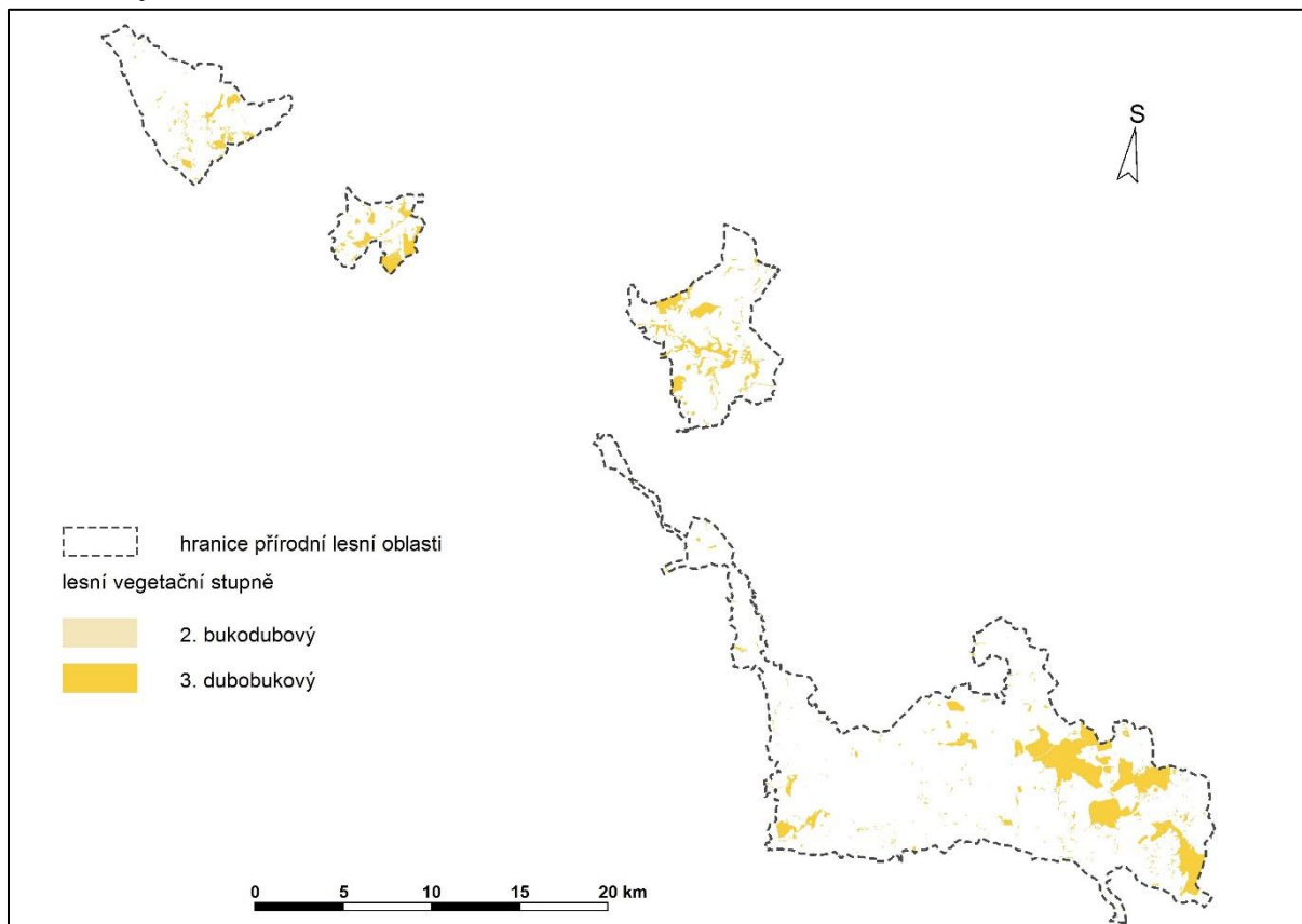
Obr. 1: Prostorová lokalizace transformovaných LVS v PLO 32 dle scénáře HadGem varianty RCP 45 i 85 v období C
