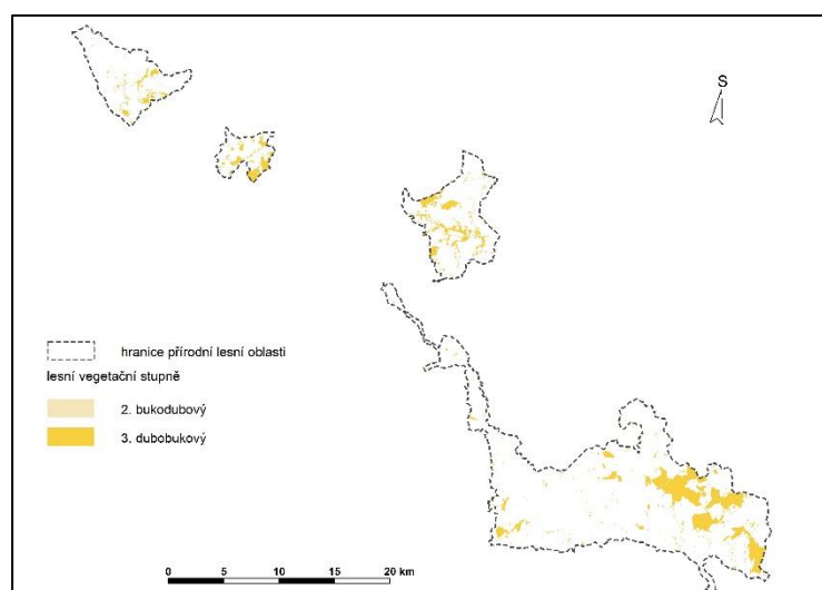
Obr. 16: Prostorová lokalizace LVS v PLO 32
