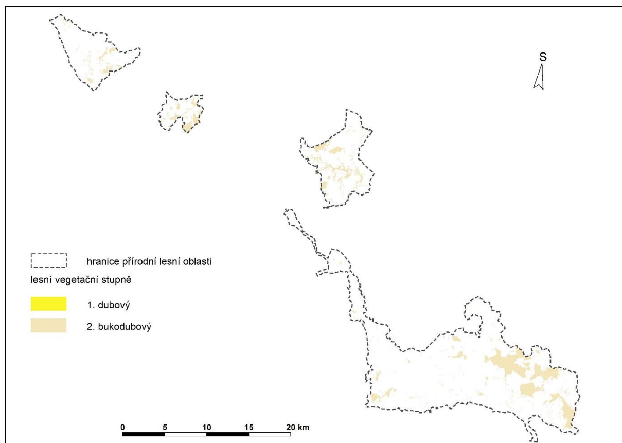
Obr. 3: Prostorová lokalizace transformovaných LVS v PLO 32 dle scénáře HadGem varianty RCP 45 v obdobích D, E a varianty RCP 85 v období D
